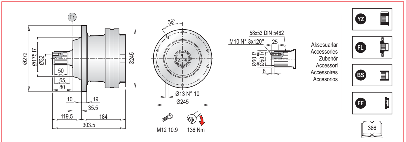
PL 5000 PS - Elektrik Motor Adaptörleri (IEC) / Electric Motor Couplings (IEC) / Anbauvorrichtung Für Elektromotore (IEC) / Predisposizioni Per Motori Elettrici (IEC) / Adaptations Pour Moteurs Electriques (IEC) / Acoplamientos Para Motores Eléctricos (IEC)
