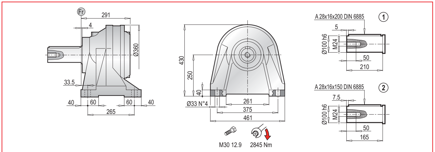
PL 16000 CPC - Elektrik Motor Adaptörleri (IEC) / Electric Motor Couplings (IEC) / Anbauvorrichtung Für Elektromotore (IEC) / Predisposizioni Per Motori Elettrici (IEC) / Adaptations Pour Moteurs Électriques (IEC) / Acoplamientos Para Motores Eléctricos (IEC)
