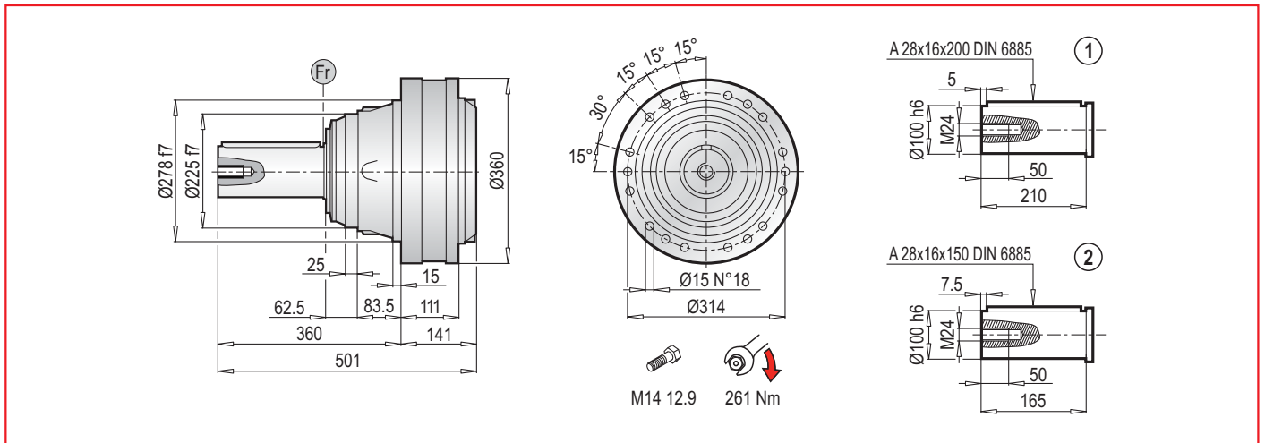
PL 16000 MC - Elektrik Motor Adaptörleri (IEC) / Electric Motor Couplings (IEC) / Anbauvorrichtung Für Elektromotore (IEC) / Predisposizioni Per Motori Elettrici (IEC) / Adaptations Pour Moteurs Electriques (IEC) / Acoplamientos Para Motores Eléctricos (IEC)
