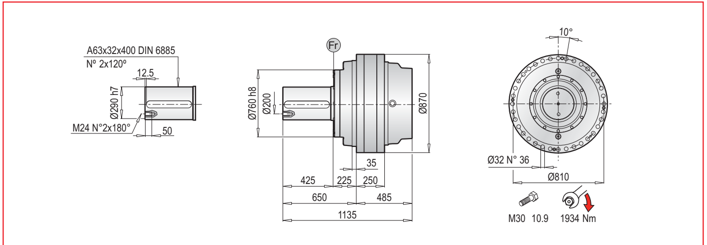
PL 300000 MC - Elektrik Motor Adaptörleri (IEC) / Electric Motor Couplings (IEC) / Anbauvorrichtung Für Elektromotore (IEC) / Predisposizioni Per Motori Elettrici (IEC) / Adaptations Pour Moteurs Electriques (IEC) / Acoplamientos Para Motores Eléctricos (IEC)
