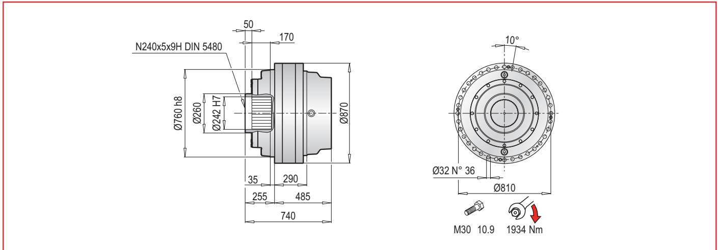
PL 30000 F - Elektrik Motor Adaptörleri (IEC) / Electric Motor Couplings (IEC) / Anbauvorrichtung Für Elektromotore (IEC) / Predisposizioni Per Motori Elettrici (IEC) / Adaptations Pour Moteurs Electriques (IEC) / Acoplamientos Para Motores Eléctricos (IEC)
