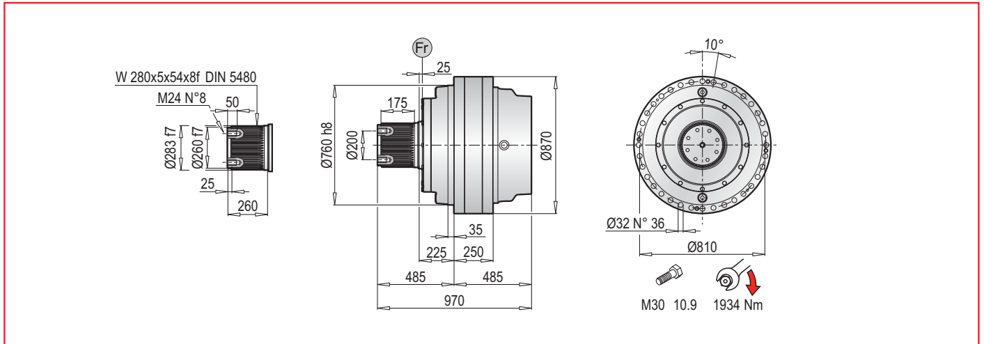
PL 300000 MS - Elektrik Motor Adaptörleri (IEC) / Electric Motor Couplings (IEC) / Anbauvorrichtung Für Elektromotore (IEC) / Predisposizioni Per Motori Elettrici (IEC) / Adaptations Pour Moteurs Electriques (IEC) / Acoplamientos Para Motores Eléctricos (IEC)
